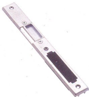
زبانه مقابل قابل ریگلاژ بزرگ کد: ۴۰۰ ۲۱۰ ۰۰۰
